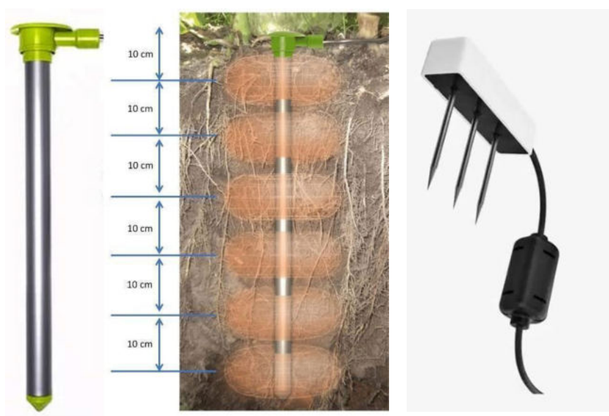
Illustration 12 : Capteur capacitif
